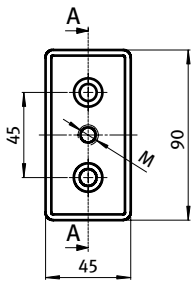
Transport- und Fußplatte 45 × 90 Transport and Base Plate 45 × 90
